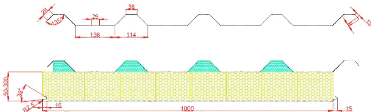
Рисунок 7. Структура Кровельной сэндвич панели.
