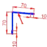
ФЭ-12. Фасонный элемент для стыковки стеновой панели с кровлей.
